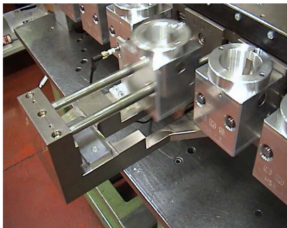
Магазин смены инструмента.
