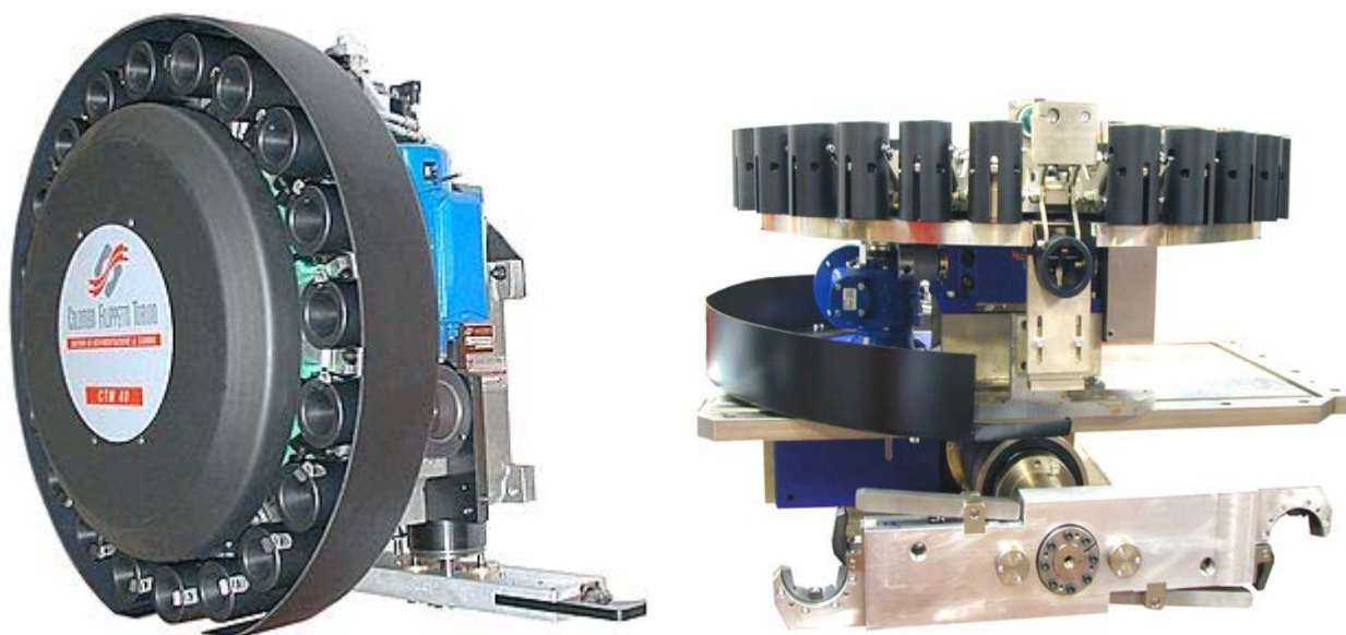
Устройства смены инструмента с магазином инструментов барабанного типа.
