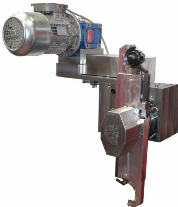
Механизм смены инструмента.
